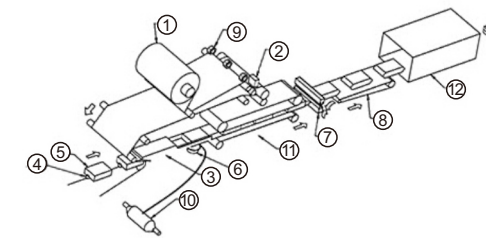
包裝流程圖
